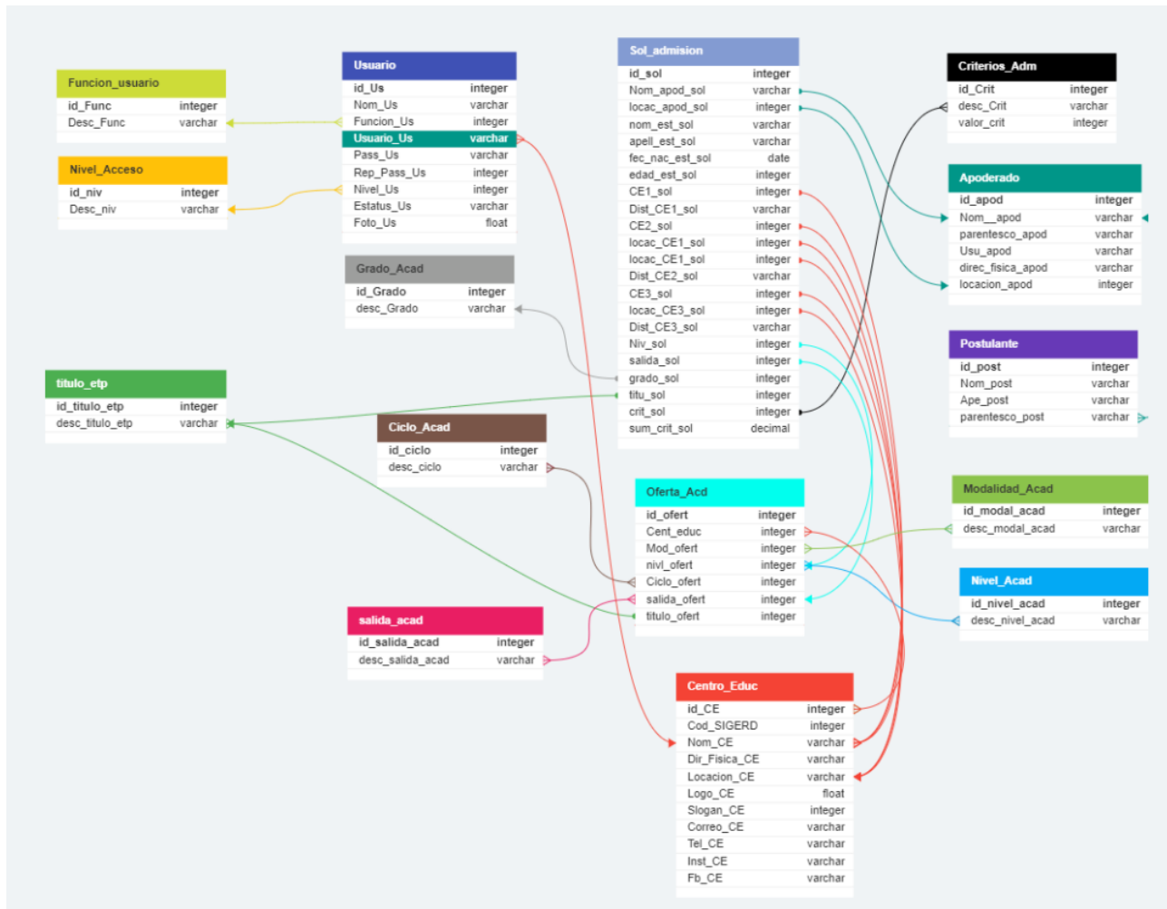
Figura 2 Diagrama Entidad-Relación
